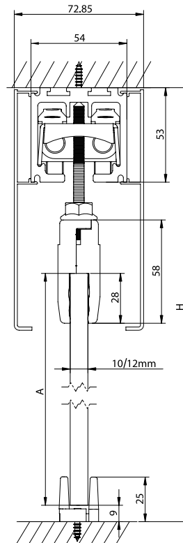
A=H-115
